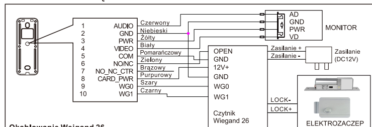
Okablowanie Weigand 26
