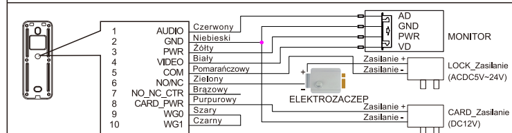
Okablowanie No
