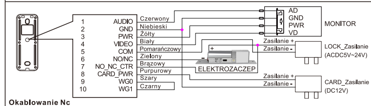
Okablowanie Nc
